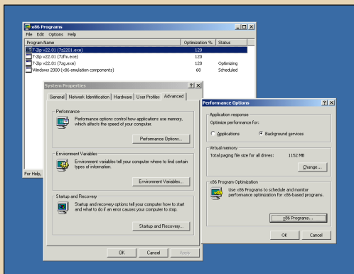
Рис. 10. Оптимизация x86-приложений в Windows 2000 for AXP реализована через интегрированную подсистему «x86 Programs»
