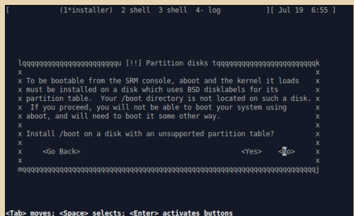
Рис. 14. Для старта Debian из SRM-консоли необходим специальный раздел для загрузчика about
