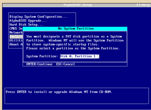
Рис. 6. Для Windows NT обязательно присутствие небольшого FAT-раздела
