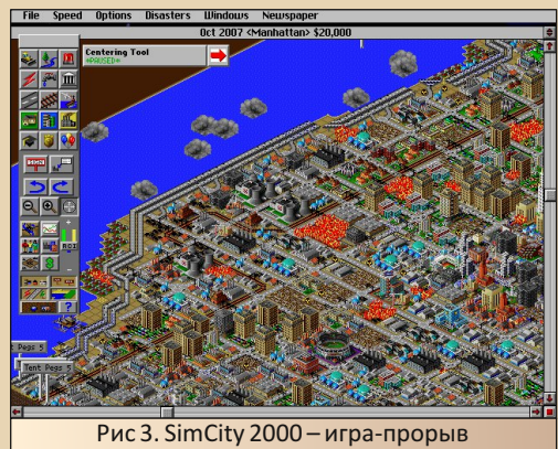
Рис 3. SimCity 2000 – игра-прорыв
