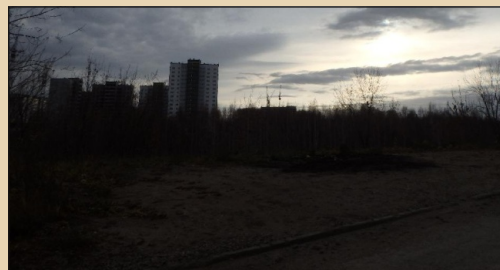
Рис. 8. Обрезанная картинка
